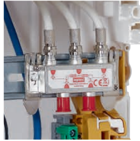
RÉPARTITEUR TV DU COFFRET BASIC
