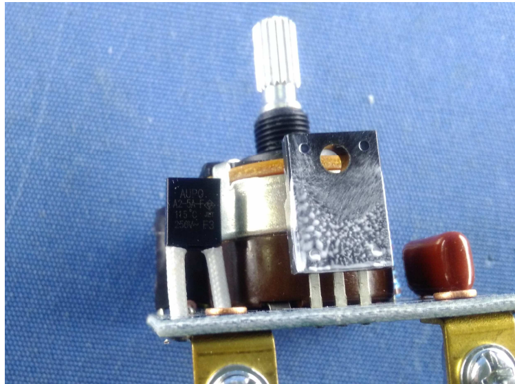
Thermal link
