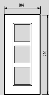
Plaque 3x2 modules entraxe 57 mm
