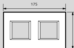
Plaque 2x2 modules entraxe 71 mm montage horizontal
