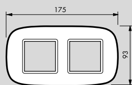
Plaque 2x2 modules entraxe 71 mm
