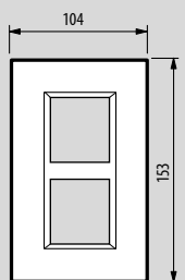
Plaque 2x2 modules entraxe 57 mm
