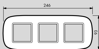
Plaque 3x2 modules entraxe 71 mm
