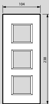
Plaque 3x2 modules entraxe 71 mm montage vertical
