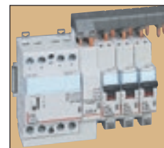
Raccordement direct par peigne d'alimentation HX 3 optimisé
